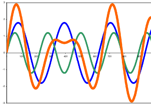
Abbildung 3: Addition zweier unkorrelierter Spannungen
