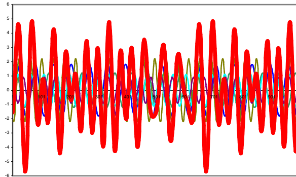
Abbildung 12: Rauschähnliches Signal mit Crestfaktor 11 dB
