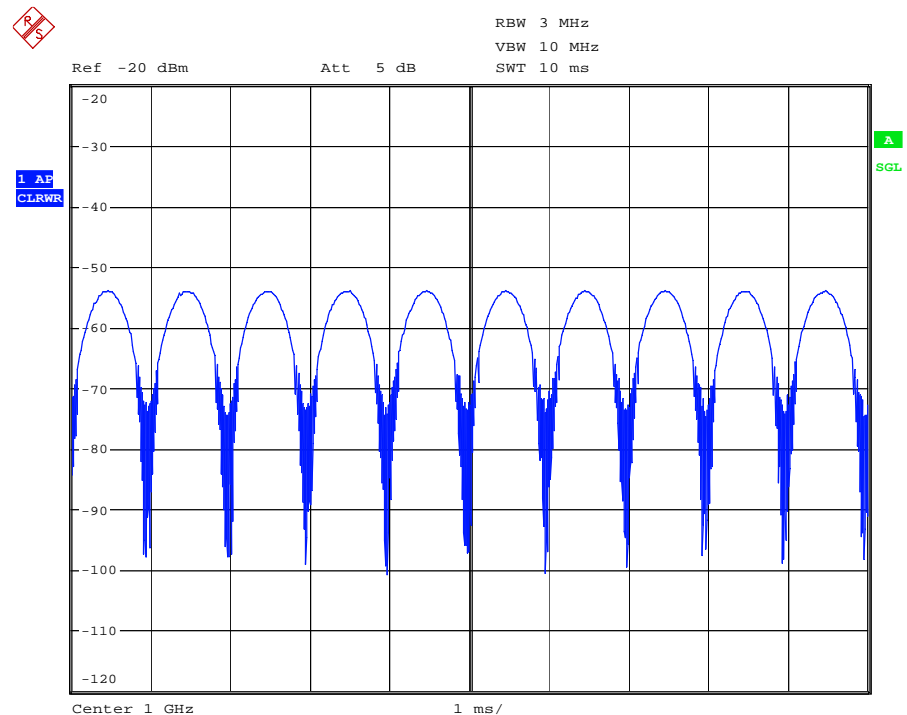
Abbildung 8: Amplitudenmoduliertes Signal
