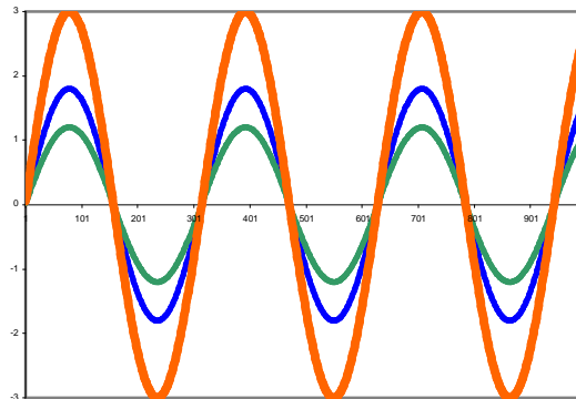
Abbildung 4: Addition zweier korrelierter Spannungen, Phasenwinkel 0^\circ Blau ist Spannung U_1 , Grün Spannung U_2 , Rot die Summenspannung U
